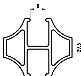
6012 (0,543 Kg/m)
