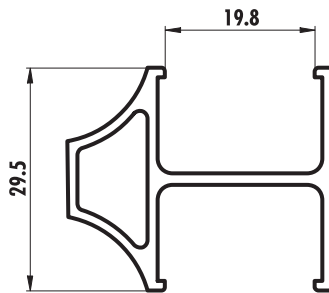
6024 (0,454 Kg/m)
