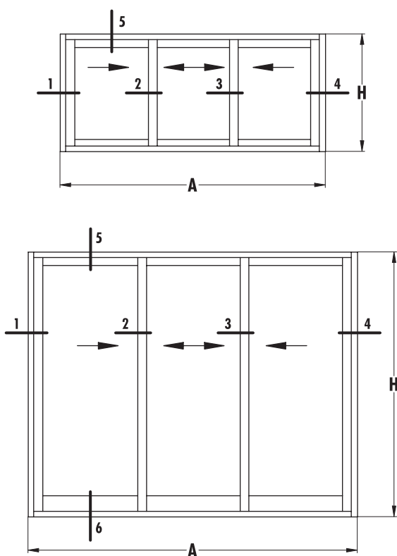
VC3 Ventana corrediza de tres hojas PC3 Puerta corrediza de tres hojas
