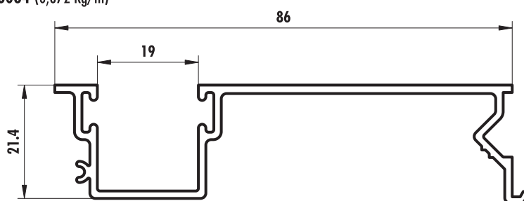
6064 (0,672 Kg/m)
