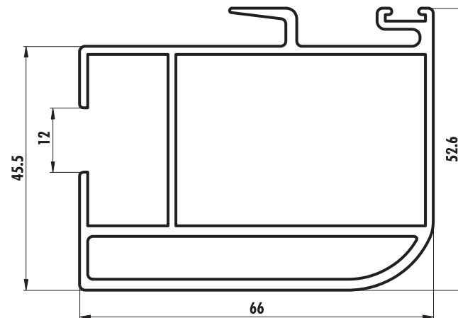
6035 (1,531 Kg/m)
