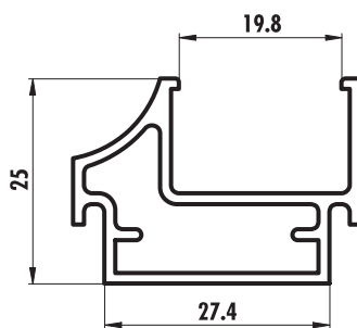
6023 (0,470 Kg/m)
