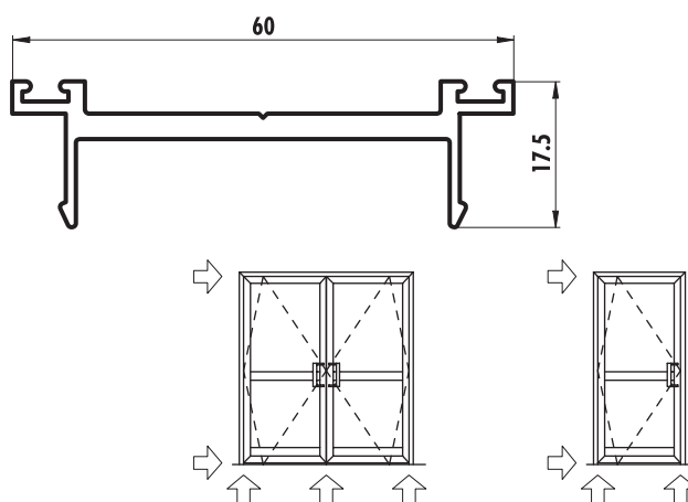
6077 (0,578 Kg/m)
