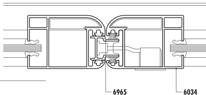
Detalle encuentro central 4 hojas
