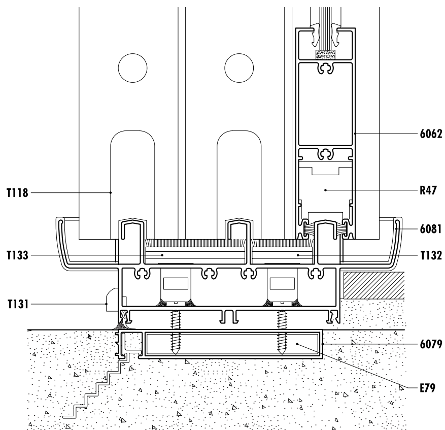
VC3 Corte 6
