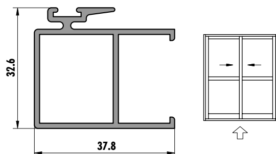
6250 (0,583 kg/m)
