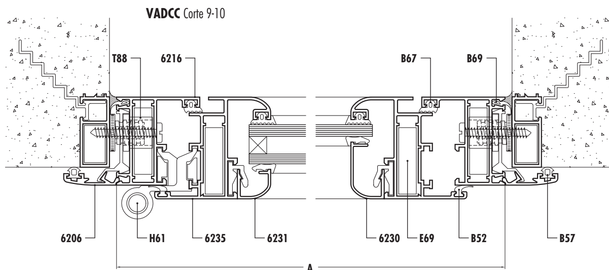
VADCR2 Corte 11-12-13
