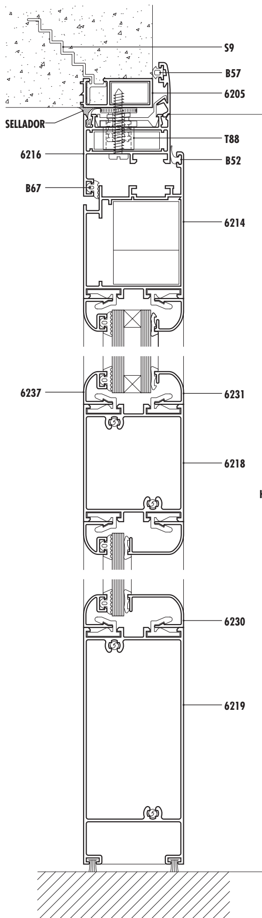
PRC Corte 1-2-3
