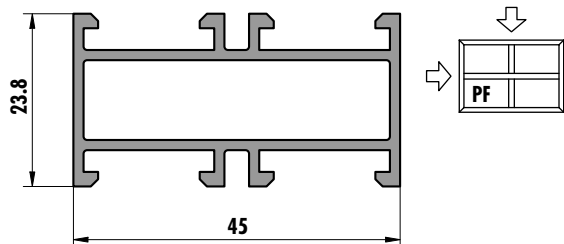
6270 (0,651 kg/m)
