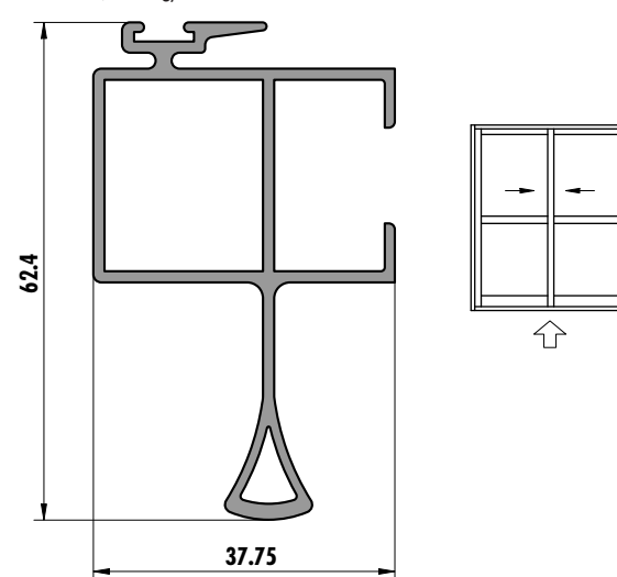
6208 (0,813 kg/m)
