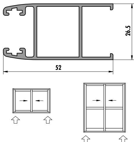
6248 (0,621 kg/m)
