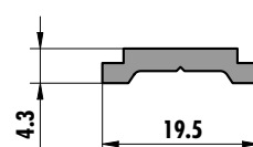
5989 (0,141 kg/m)
