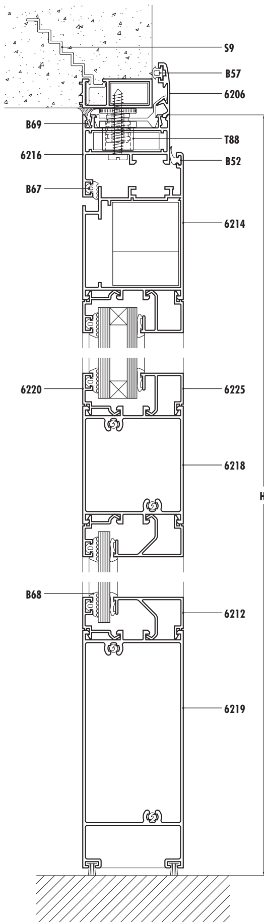
PRR Corte 1-2-3
