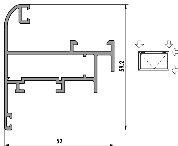
6236 (0,907 kg/m)
