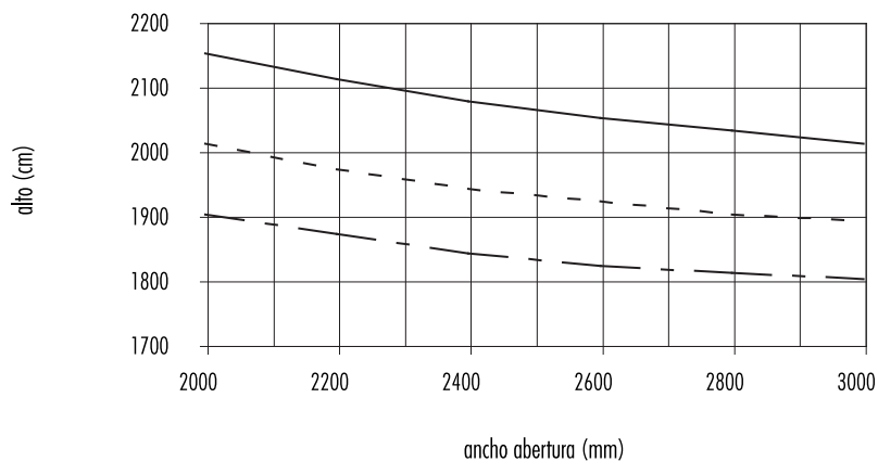
Parante central 6908-6910
