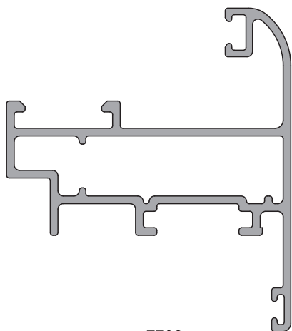
7708 0,902 kg/m
