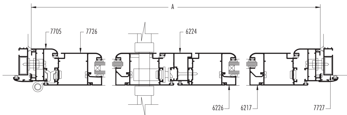
SECCION 1-2-3
