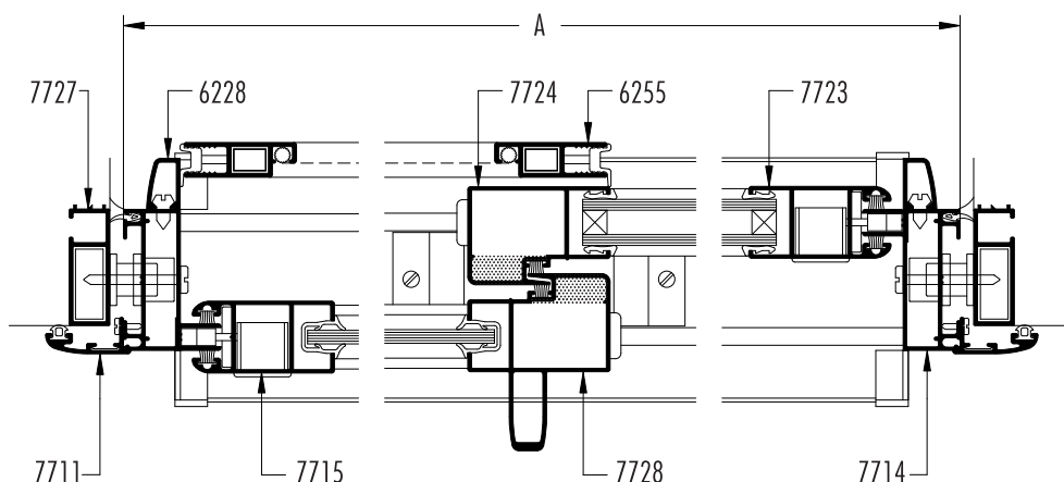
SECCION 1-6-3
