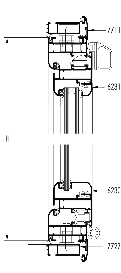
SECCION 3-4
