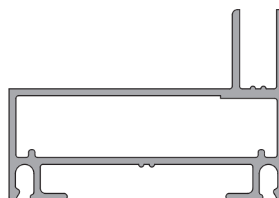
7714 0,724 kg/m
