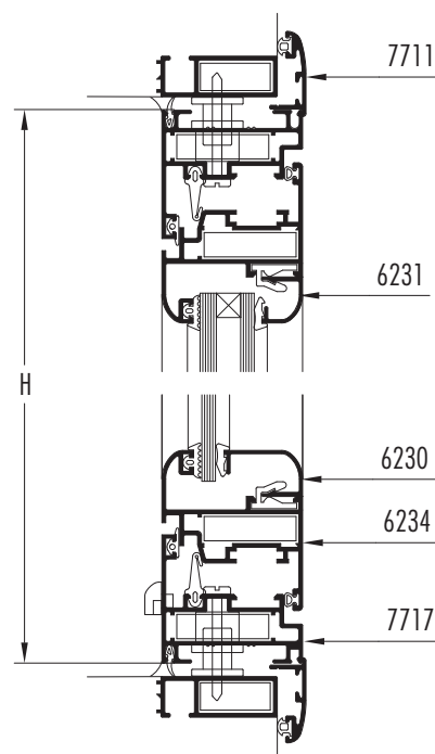
SECCION 3-4
