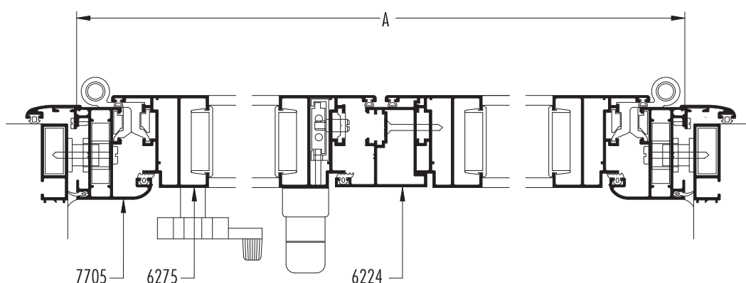
SECCION 1-2-3
