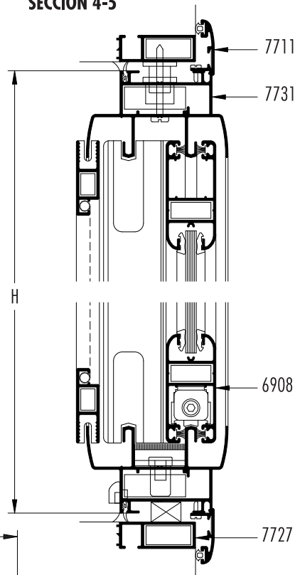
SECCION 4-5
