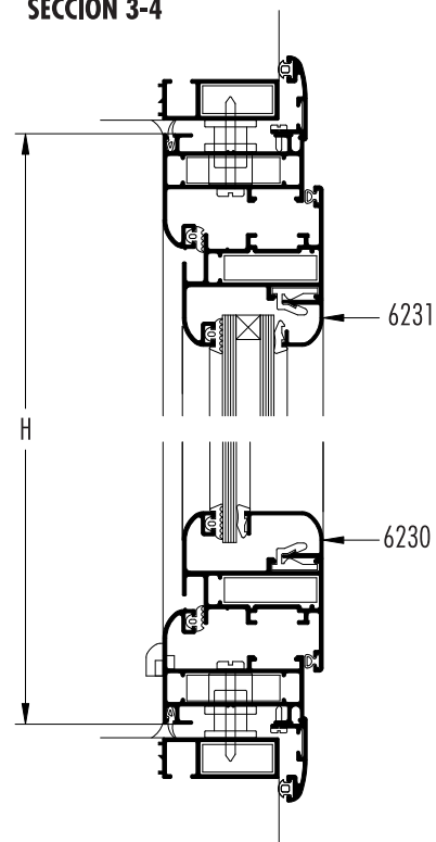
SECCION 3-4
