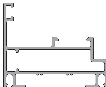
7707 0,772 kg/m
