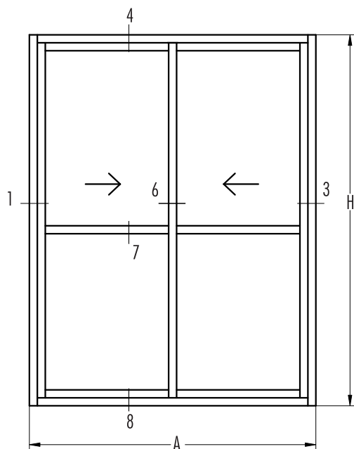
SECCION 1-6-3
