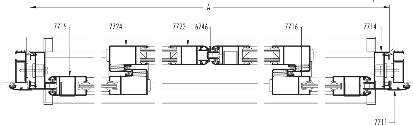
SECCION 1-2-3-4
