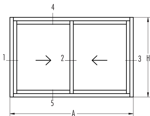
SECCION 1-2-3
