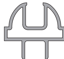
6267 0,383 kg/m
