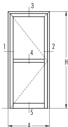
SECCION 1-2
