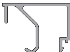
6217 0,294 kg/m
