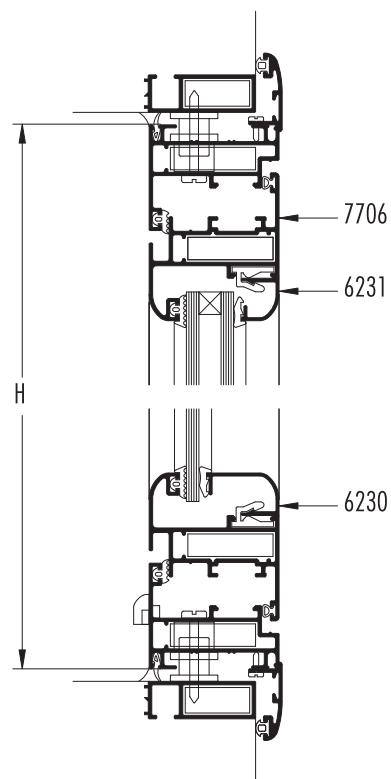
SECCION 3-4
