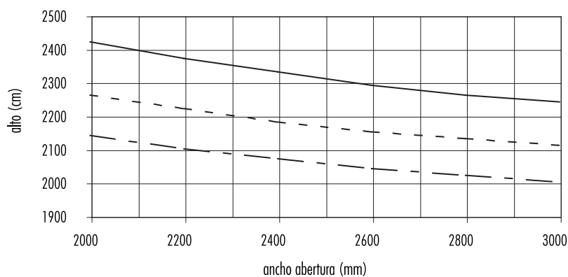
Parante central 6910-6910
