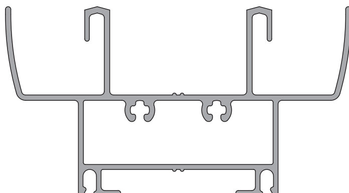
7713 1,310 kg/m
