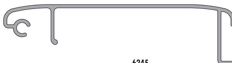
6245 0,629 kg/m
