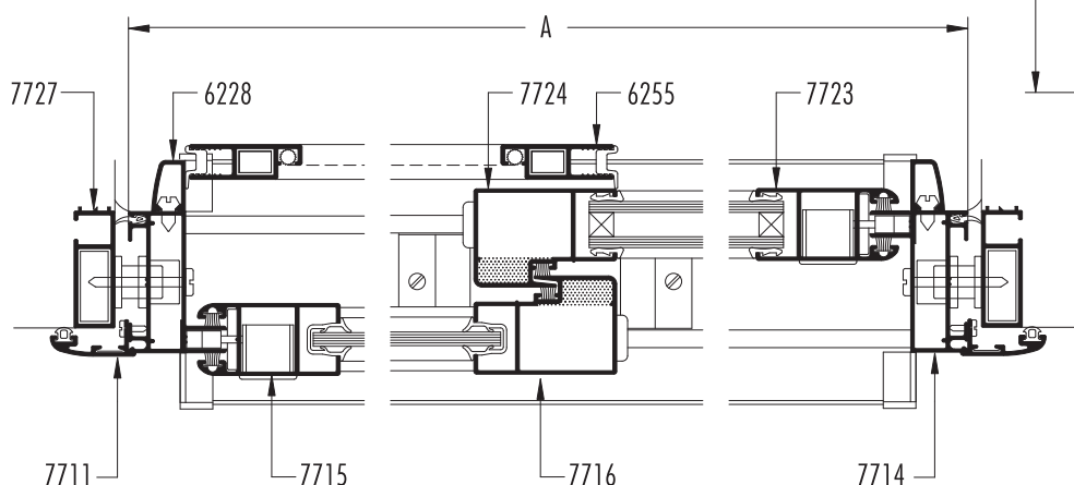
SECCION 1-2-3
