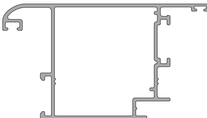
7877 1.185 kg/m
