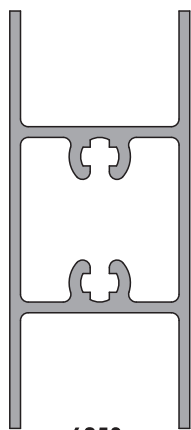
6253 0,689 kg/m
