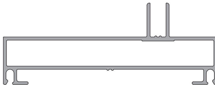
8008 1.066 kg/m
