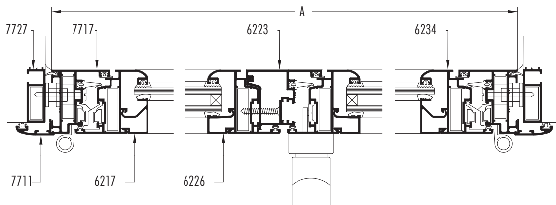
SECCION 1-5-6
