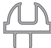
6266 0,383 kg/m
