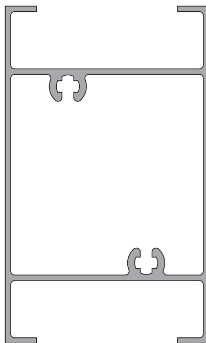
6276 1,301 kg/m
