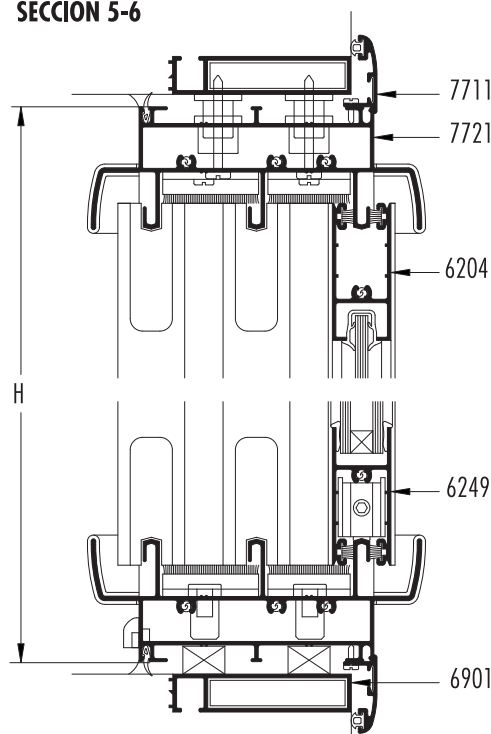
SECCION 5-6
