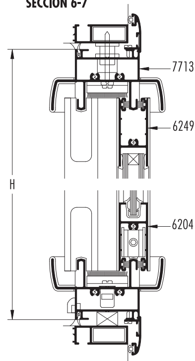
SECCION 6-7
