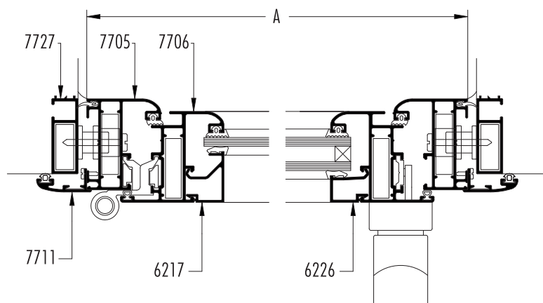
SECCION 1-2
