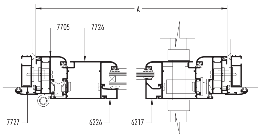
SECCION 1-2
