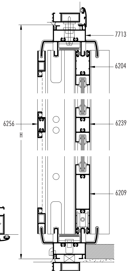
SECCION 4-7-8
