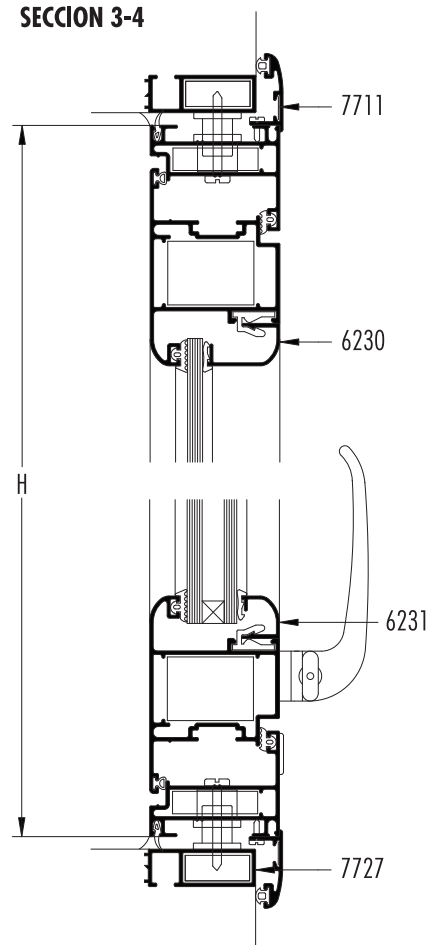
SECCION 3-4
