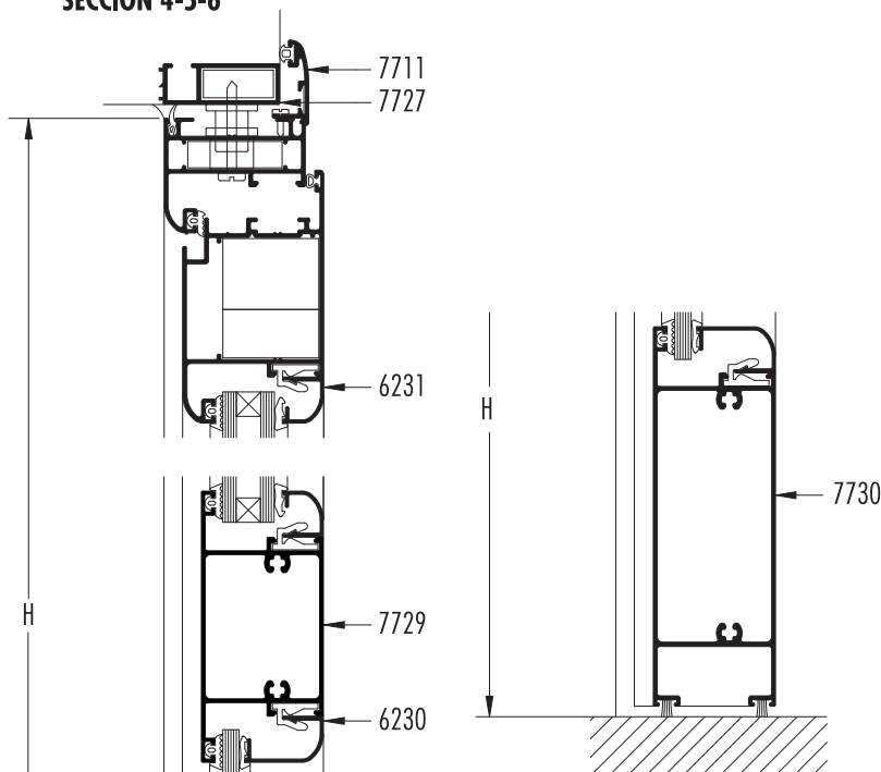
SECCION 4-5-6
