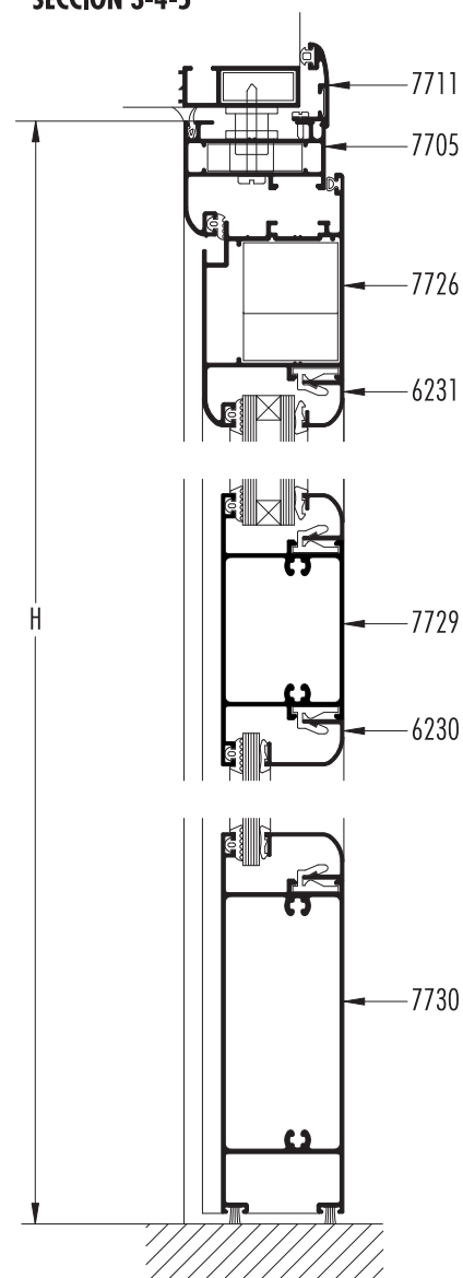
SECCION 3-4-5
