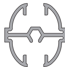
6268 0,429 kg/m
