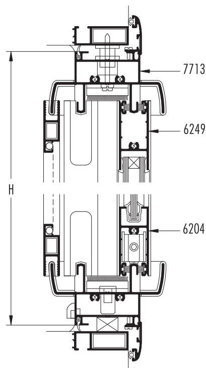
SECCION 4-5
