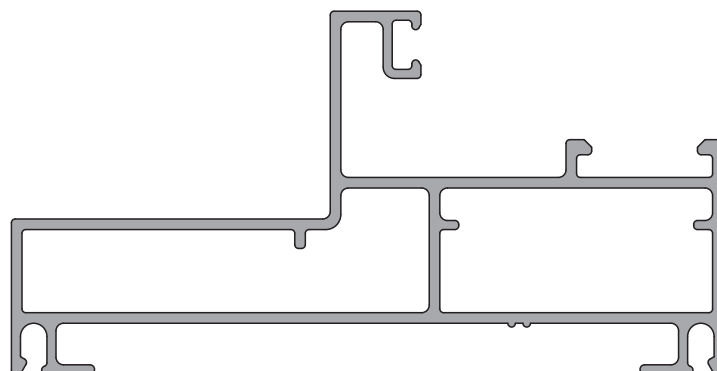
8010 1.291 kg/m
